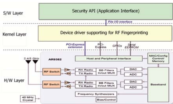
(그림 7) 변복조 특성 기반 RF 핑거프린트 플랫폼 구조
