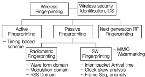
(그림 3) 무선 핑거프린팅 방식 분류
