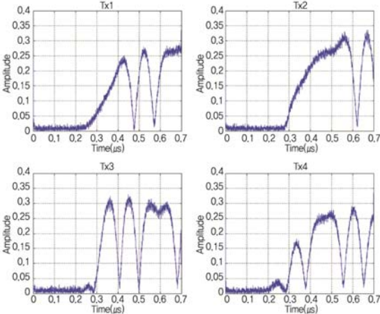
(그림 5) 과도파 구간과 4개의 무선랜 NIC(동일 제조사/모델)에 대한 과도파 동작패턴 예제[6]
