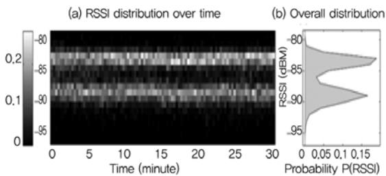
(그림 8) 동일위치-시간변화에 따른 RSS 분포[9]
