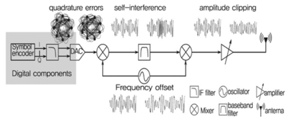
(a) RF 송신기 HW단에서의 제작 허용오류 유형
