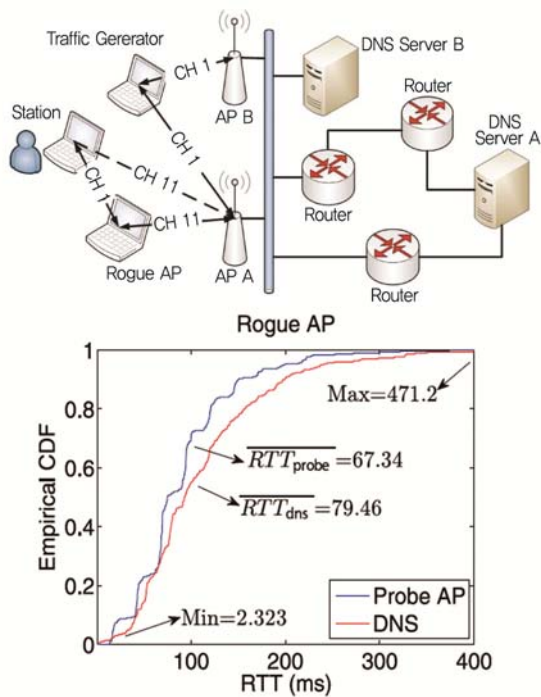
(그림 4) 클론AP 공격환경 및 평균 RTT 기반 복제/위장AP 탐지[3]
