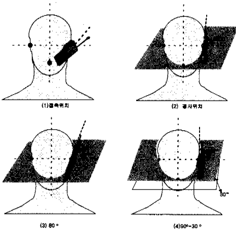
그림 2. 휴대전화에 대한 전자파흡수를 시험위치 Fig. 2. SAR test position of mobile phone.
