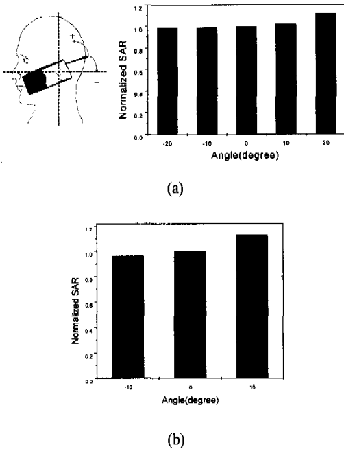
그림 5. 접촉위치와 경사위치에서의 회전에 따른 전자파흡수율 비교. (a) 접촉위치, (b) 경사위치 Fig. 5. Comparison of SAR value for rotation of mobile phone at touch and tilt position. (a) touch position, (b) tilt position.
