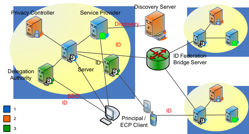
( 4) e-IDMS
