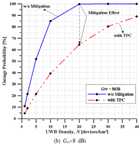
그림 4. WiMAX의 outage. Fig. 4. Outage in WiMAX.
