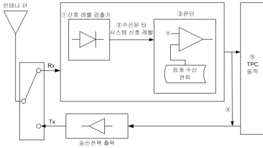
그림 3. UWB 시스템의 TPC 동작도 Fig. 3. Diagram of TPC operation in UWB system.
