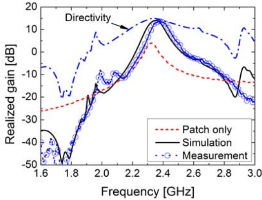
그림 9. 와이브로 안테나의 실현 이득 및 지향 특성 ( d=72 mm, w_s=242 mm, \Theta=\phi=0 )
