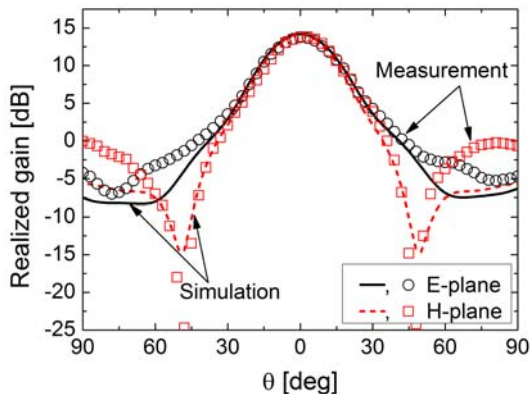
그림 10. 와이브로 안테나의 복사 패턴( f=2.35 GHz) Fig. 10. Radiation patterns of the Wipro antenna( f=2.35 GHz).
