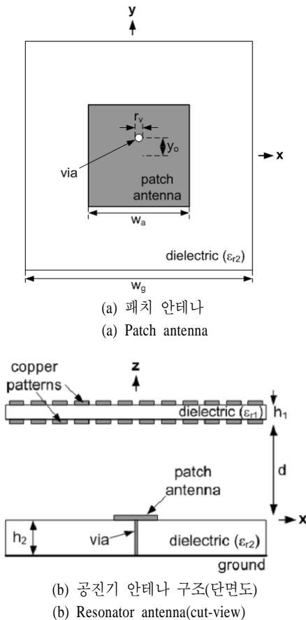
그림 5. 공진기 안테나 및 피더로 사용된 패치 안테나 구조( r_v=1.0 mm, y_o=4 mm, h_2=1.52 mm, w_a=32.5 mm, w_g=262 mm, \epsilon_{r1}=6.15 , \epsilon_{r2}=3.5 ) Fig. 5. Geometry of a resonator antenna and a patch antenna( r_v=1.0 mm, y_o=4 mm, h_2=1.52 mm, w_a=32.5 mm, w_g=262 mm, \epsilon_{r1}=6.15 , \epsilon_{r2}=3.5 ).
