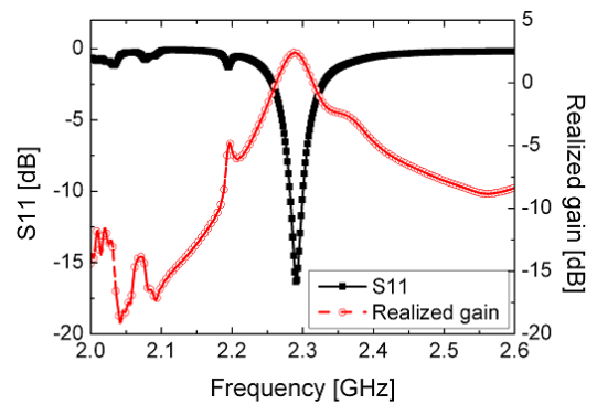
그림 6. 메타 물질 상부 덮개로 덮여 있으며 작은 접지면을 갖는 안테나의 특성( d=2 mm, w_g=50 mm, \Theta=\Phi=0 ) Fig. 6. Behaviors of the antenna with a small ground plane, which is covered with metamaterial superstrate( d=2 mm, w_g=50 mm, \Theta=\Phi=0 ).
