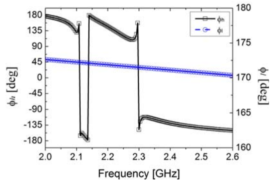
그림 7. 메타 물질 상부와 접지면의 반사 위상 Fig. 7. Reflection phases of the metamaterial superstrate and ground substrate.
