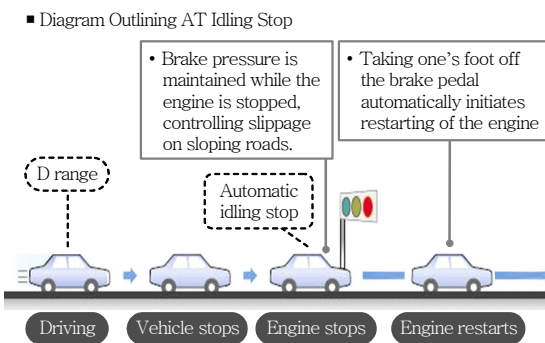
(그림 2) Stop-Start 시스템 작동 원리
