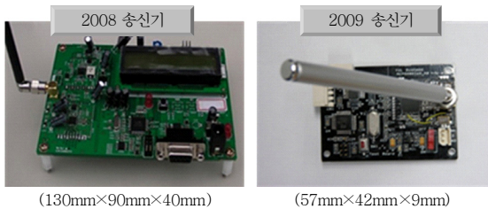
(그림 5) 2008 송신기와 2009 송신기 비교
