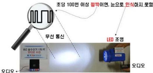
[그림 2] 가시광 무선 통신의 원리
