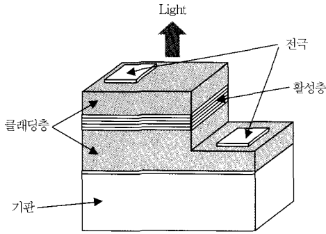
(그림 10) 일반형 LED 칩의 개요도
