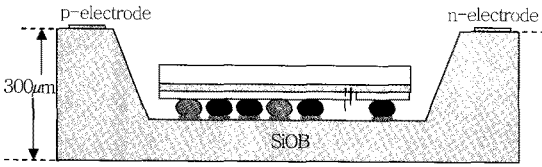
(그림 29) Si based WPL
