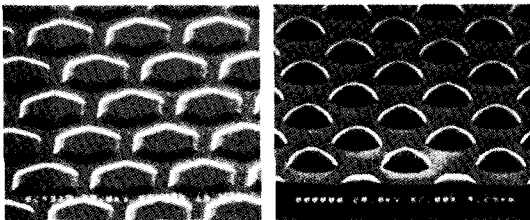
(그림 16) PSS 표면 가공 모습
