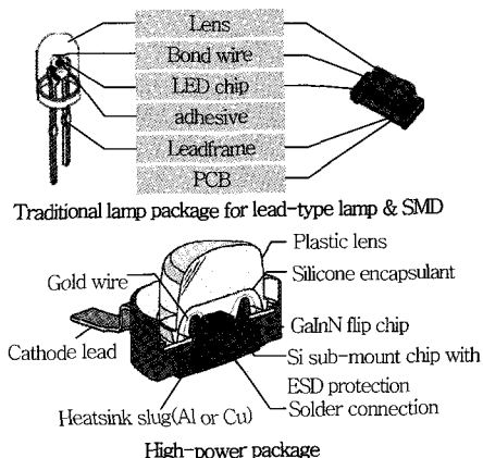
(그림 21) LED 패키지
