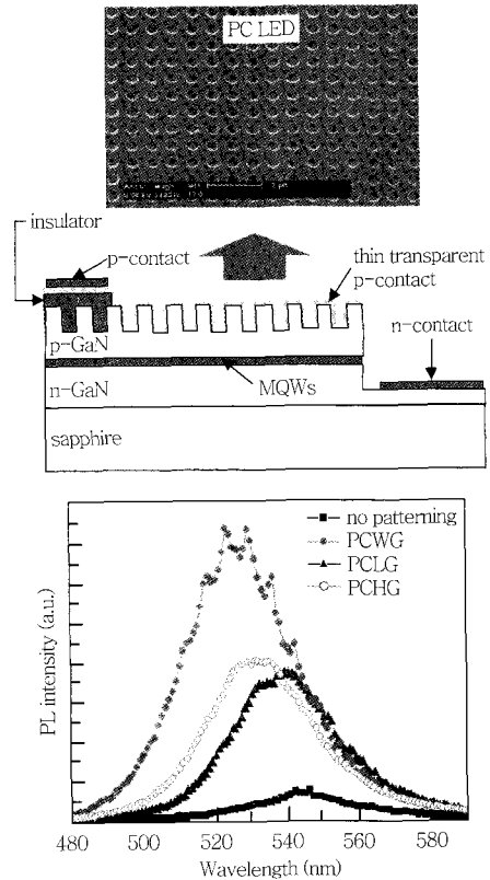
(그림 18) PBC의 구조 및 발광 효율의 향상
