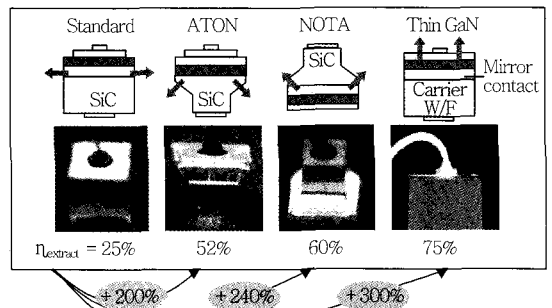
(그림 13) SiC LED 칩의 구조 변화
