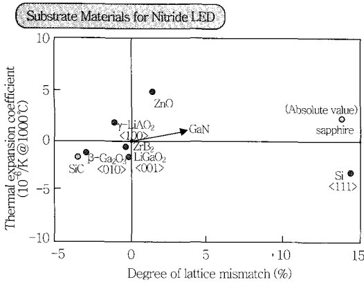
(그림 2) 기판 재료의 격자 불일치 정도와 열팽창 계수
