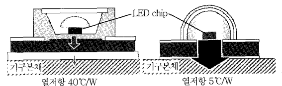
(그림 28) COB 패키지
