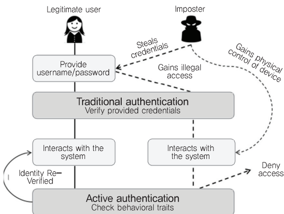
(그림 1) 기존 인증과 무자각 지속인증의 차이점
