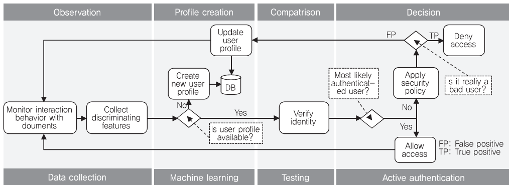
(그림 2) 무자각 지속인증의 기본 프로토콜
