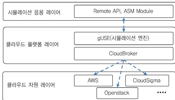
(그림 3) CloudSME 시뮬레이션 플랫폼
