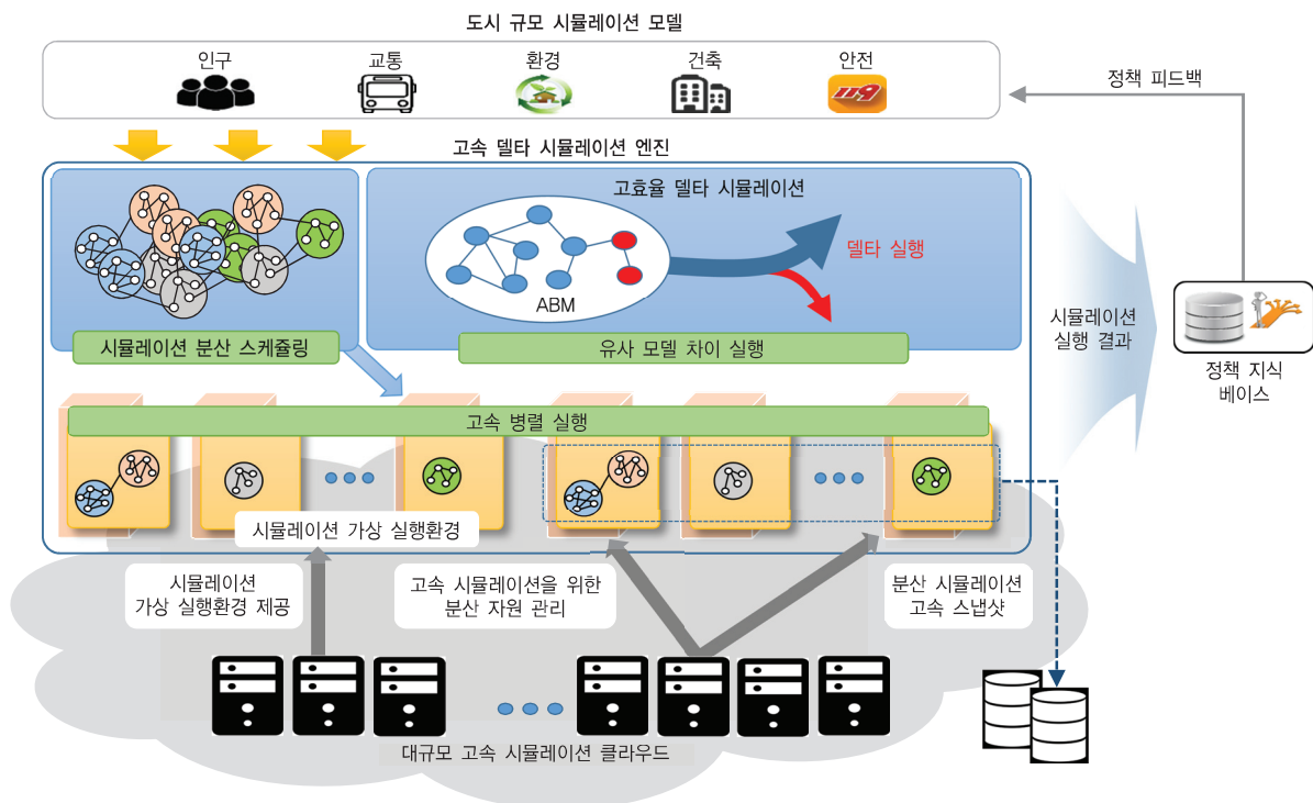
(그림 5) 클라우드 기반 고속 시뮬레이션 개념도
