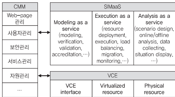
(그림 1) CSim 구조
