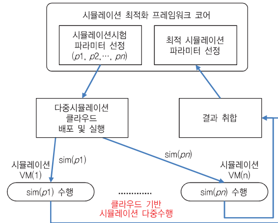
(그림 4) 시뮬레이션 최적화 프레임워크
