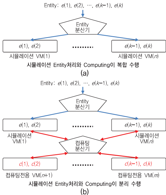
(그림 2) CSim의 시뮬레이션 실행 방식: (a) 전통적 모델, (b) 제안된 모델
