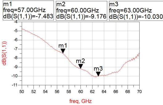
그림 13. RF 포트 정합 특성 Fig. 13. Impedance matching to RF port.
