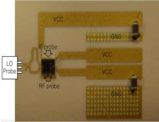
그림 8. 측정 기판 Fig. 8. Ceramic substrate for measurements.
