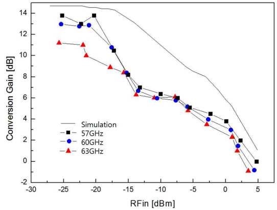
그림 11. 하향 변환 혼합기 변환 이득 Fig. 11. Conversion gain of down conversion mixer.
