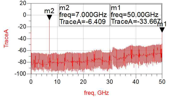
그림 10. IF&LO 특성(RF: 57 GHz -20.28 dBm, LO: 50 GHz +0.12 dBm) Fig. 10. Characteristics of IF&LO(RF: 57 GHz -20.28 dBm, LO: 50 GHz +0.12 dBm).
