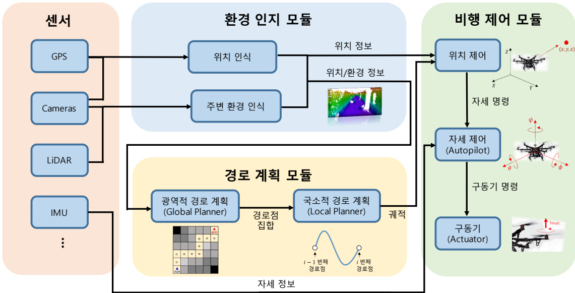
그림 1 무인 비행체의 자율 비행을 위한 환경 인지 및 경로 계획 구성도
