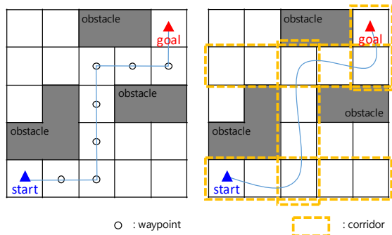
그림 3 경로점 기반 path planning(왼쪽)과 corridor 기반 path planning(오른쪽)
