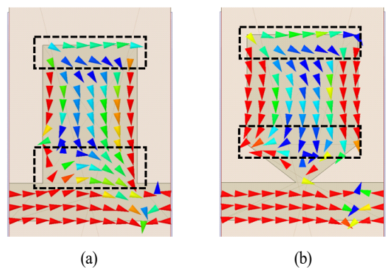
그림 6. (a) 기존 방사소자와 (b) 제안한 방사소자의 전류분포 Fig. 6. Electric current distribution of (a) conventional and (b) proposed radiating element.
