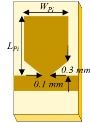
그림 5. 제안한 방사소자의 단위 셀 Fig. 5. Unit cell of proposed radiating element.
