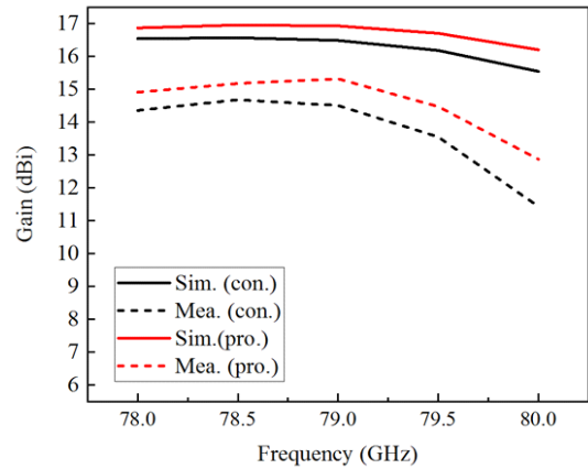
그림 10. 안테나 정면에서의 주파수에 따른 이득 변화
