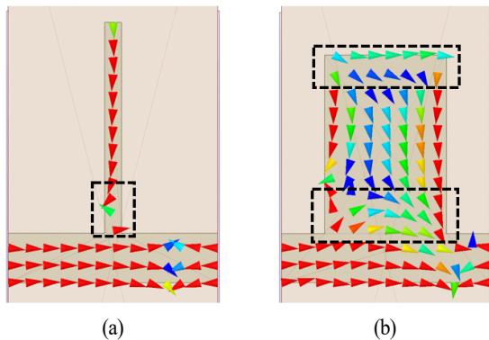
그림 4. (a) 폭이 좁은 방사소자와 (b) 폭이 넓은 방사소자의 전류분포 Fig. 4. Electric current distribution of (a) narrow and (b) wide radiation elements.
