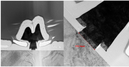
그림 6 0.18 \mu\text{m} 게이트 길이를 갖는 GaN HEMT 게이트 구조
