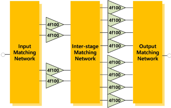
그림 8 28GHz 전력증폭기 회로 구성도
