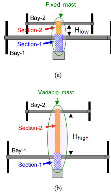
그림 3. 높이 가변형 멀티 베이 배열 안테나 Fig. 3. Adjustable height multi-bay array antenna.
