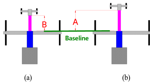
그림 4. 높이 가변형 안테나 형상 Fig. 4. Height-adjustable mast antenna configuration.
